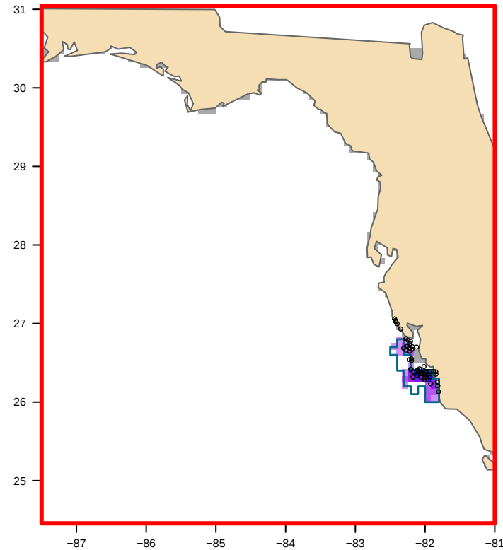
USED: VIIRS-clipped (21 positive VIIRS cells) bloom area 2,222 km 2
