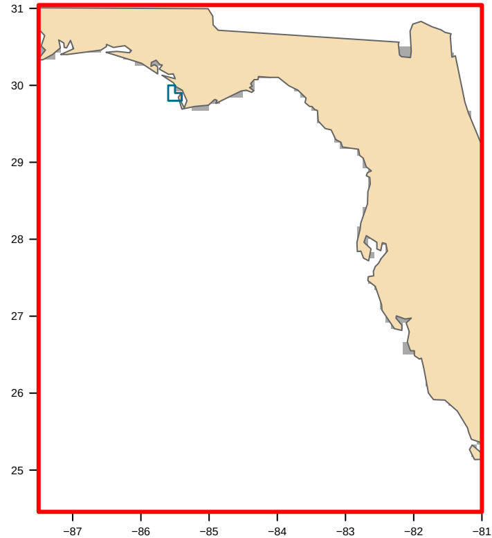
USED: VIIRS-clipped (3 positive VIIRS cells) bloom area 0 km2
