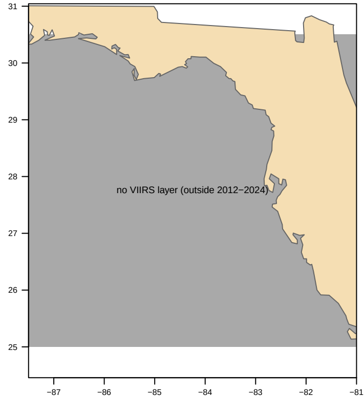
VIIRS-clipped
