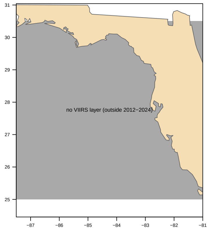
VIIRS-clipped
