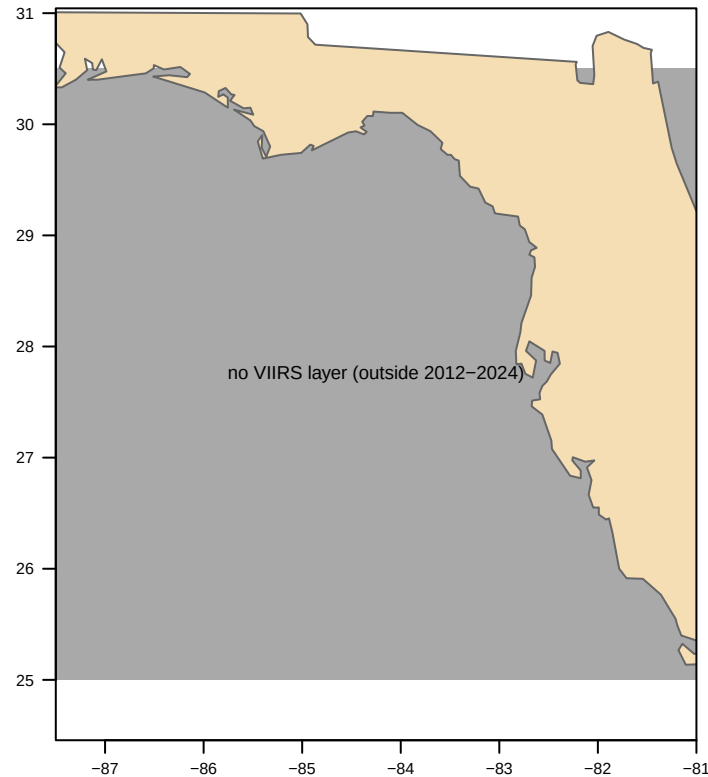
VIIRS-clipped
