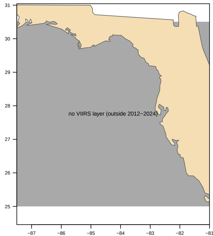
VIIRS-clipped
