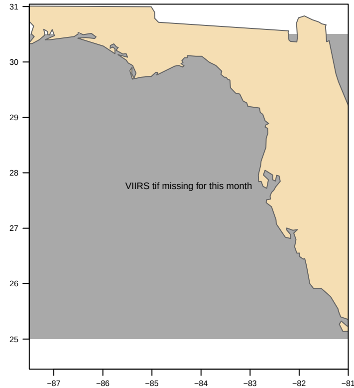
VIIRS-clipped
