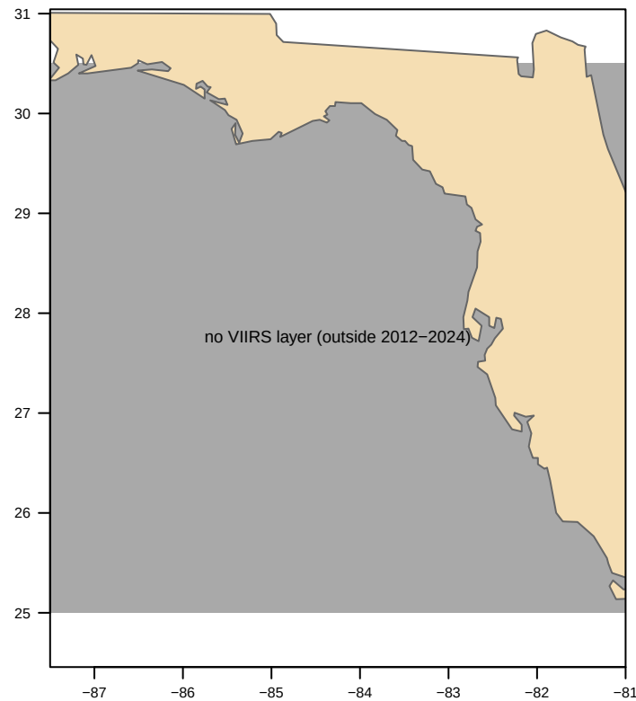
VIIRS-clipped
