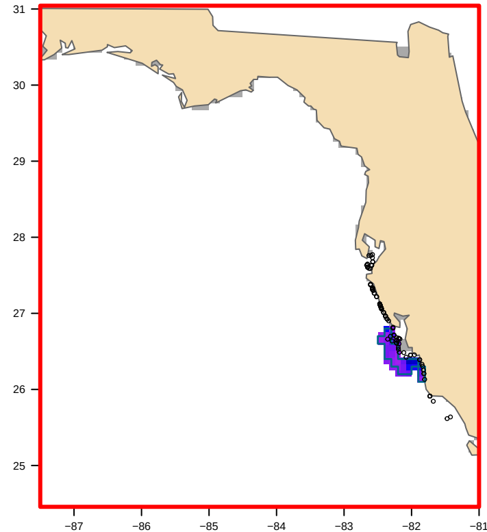
USED: VIIRS-clipped (15 positive VIIRS cells) bloom area 2,527 km 2
