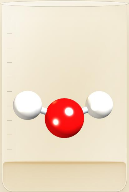
水 Water H 2 O
