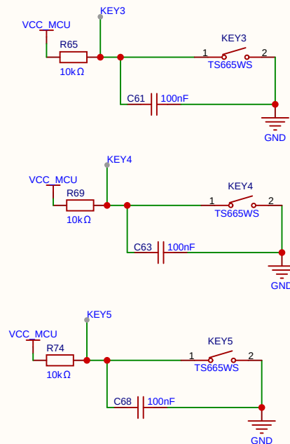
按键模块
