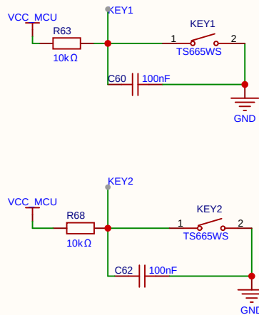
按键模块
