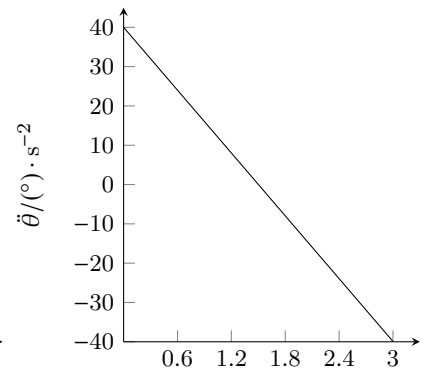
(c) 角加速度
