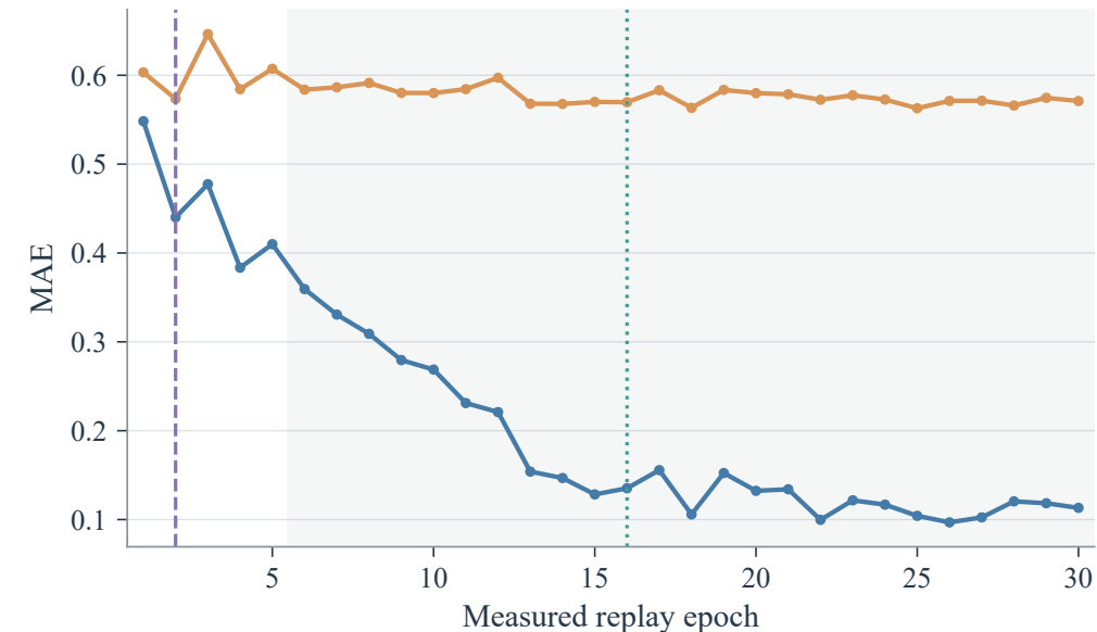
(d) MAE
