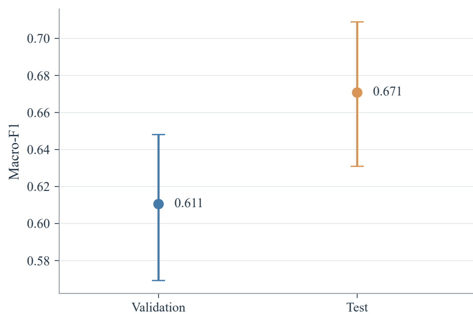
(b) Macro-F1
