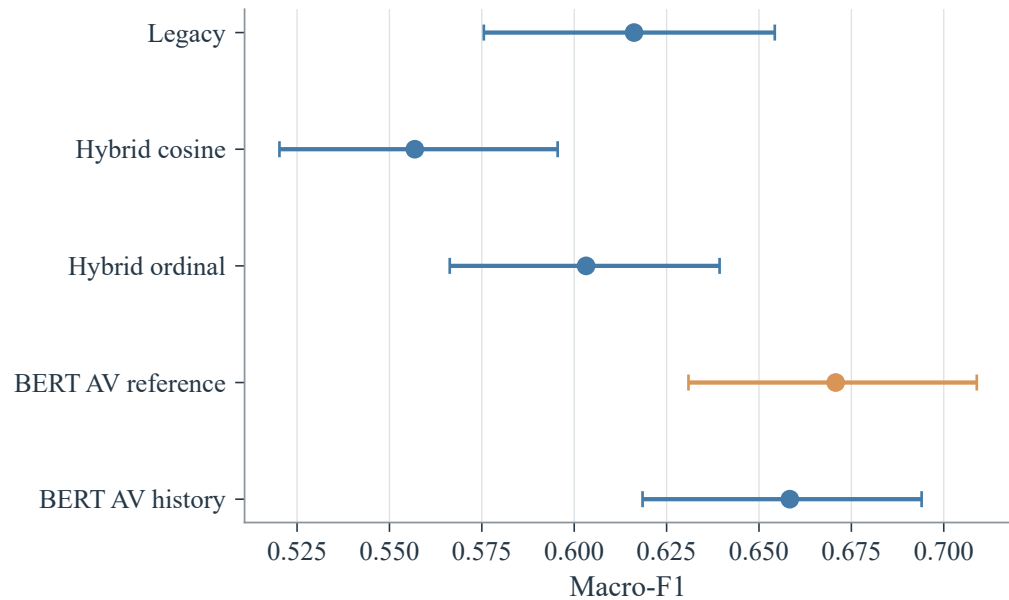
(b) Macro-F1
