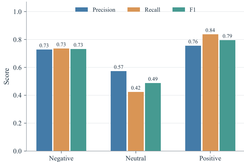
(b) Test
