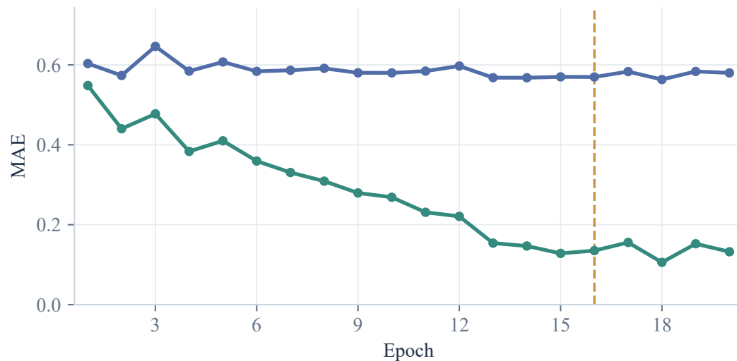
(d) Regression error
