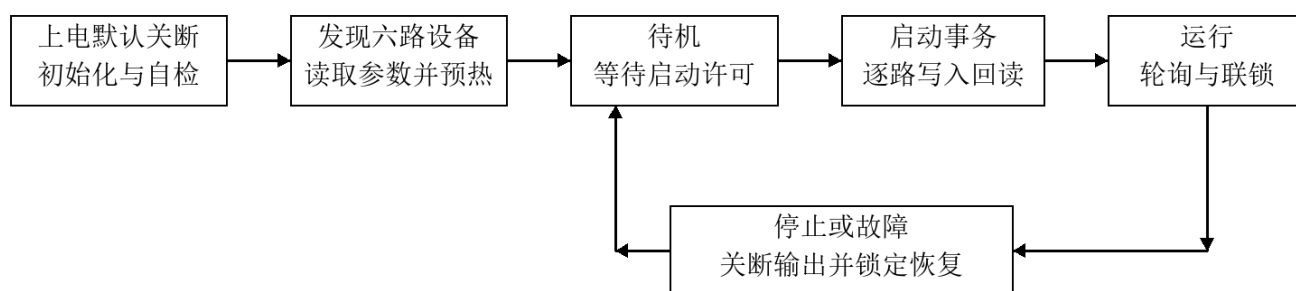
图 3-2 软件总体运行流程
