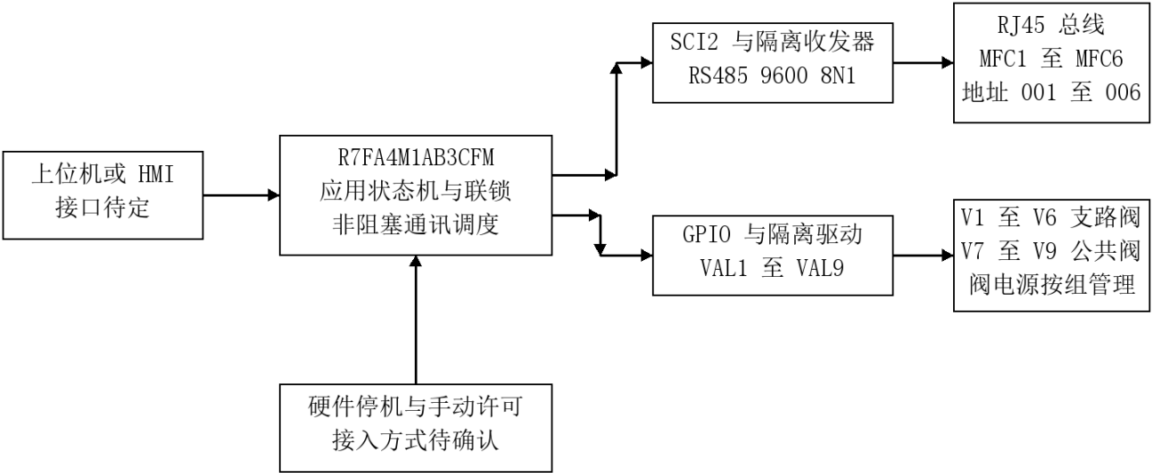
图 3-1 硬件功能框图
