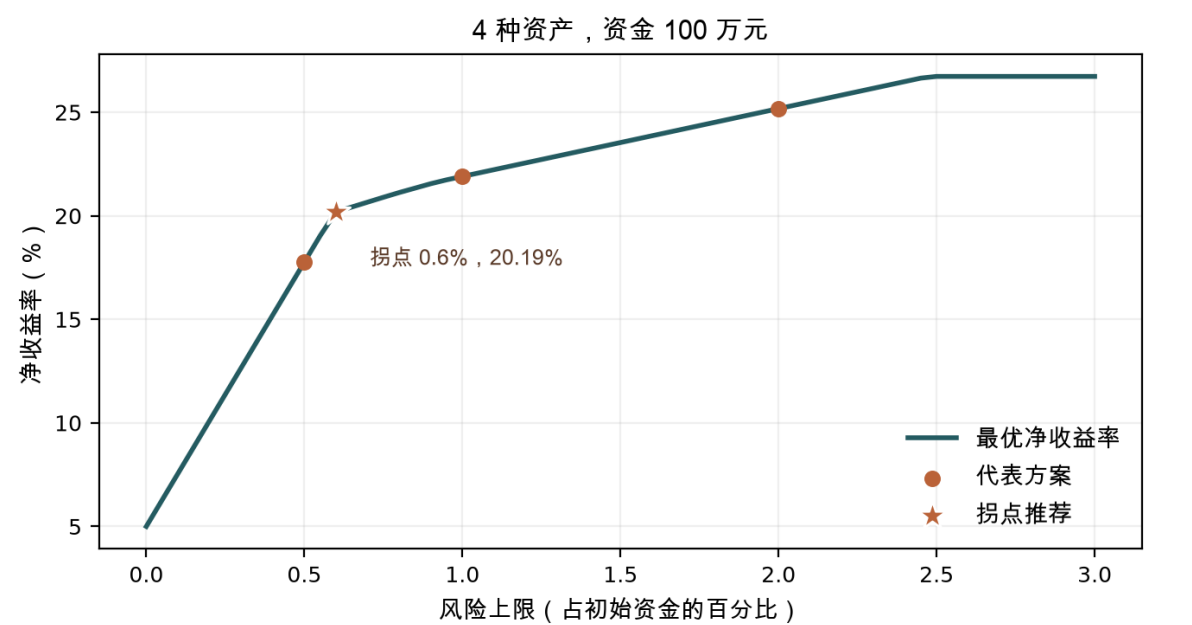
图 1 四资产风险上限与最优净收益率；圆点为代表方案，星号为拐点推荐（第 8 节），横轴为约束上限。
