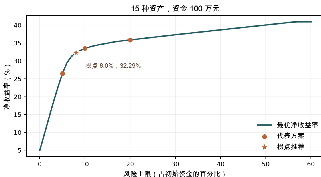
图 2 十五资产最优收益包络；圆点为代表方案，星号为拐点推荐（第 8 节），平台区不表示风险上限全部被用尽。
