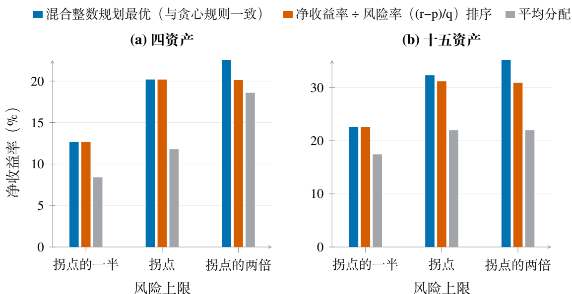
图4 简单规则与最优方案的差距
