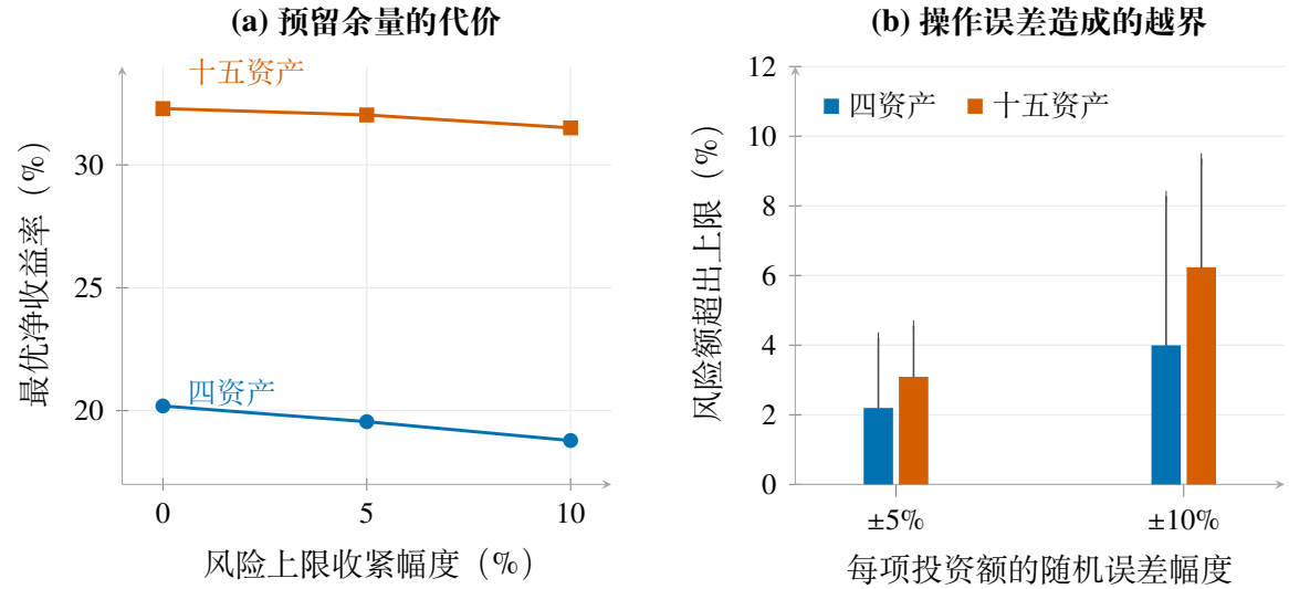
图3 安全余量的代价与操作误差的危害
