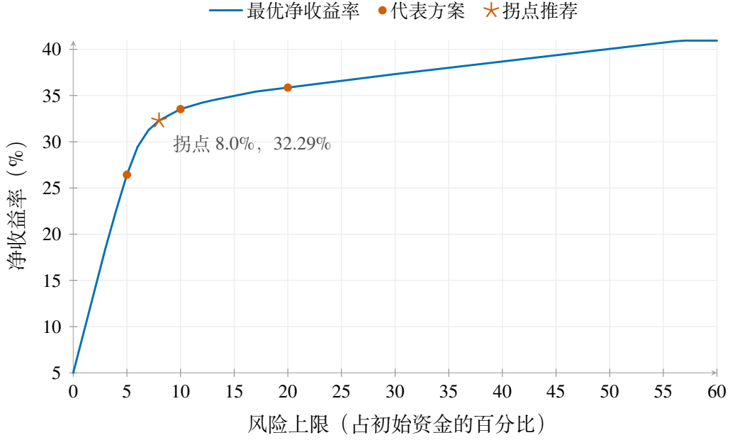
图2 十五资产最优收益包络
