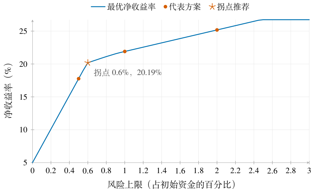
图1 四资产风险上限与最优净收益率
