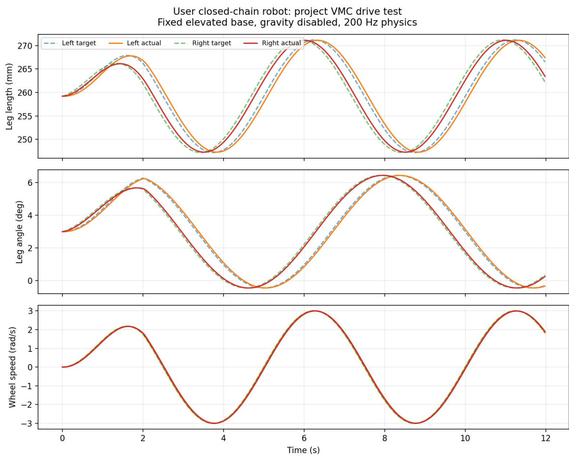
图 6 悬空 VMC 的目标与实际跟随 这是机械与控制映射验证
