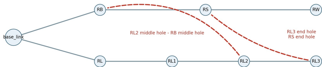
图 2 右腿拓扑变化 实线为原关节树 红色虚线为新增约束 左侧完全镜像
