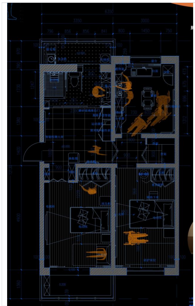
01改造后平面布置（带尺寸）
