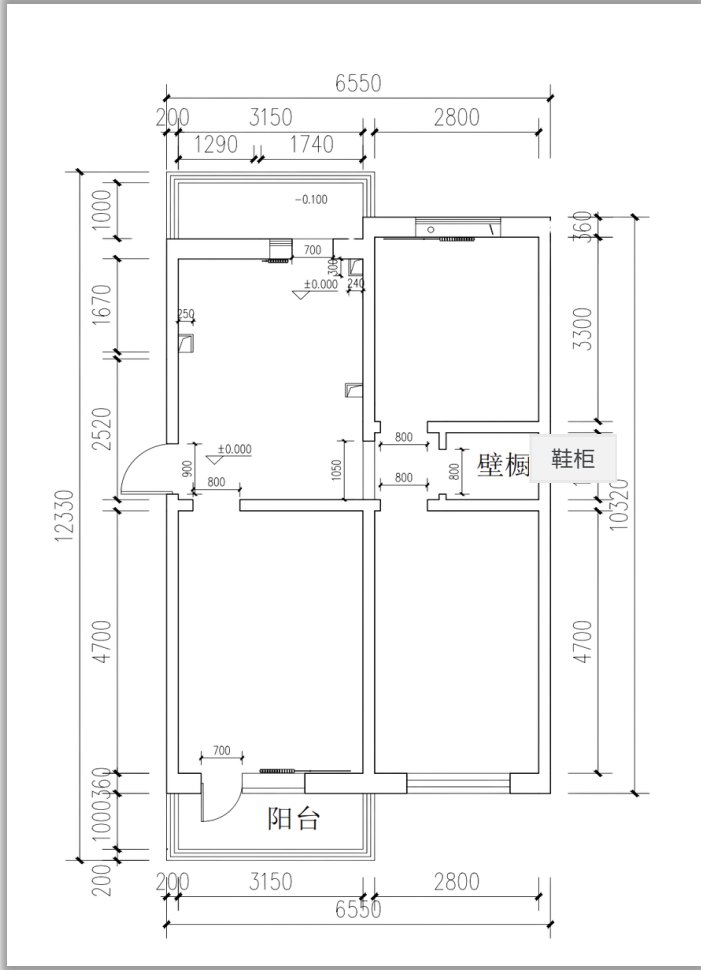
02-清理后平面 (带尺寸)
