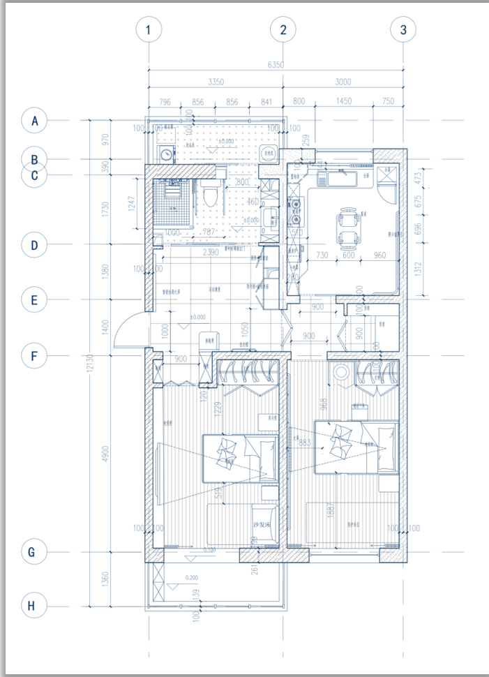
03-改造后平面布置 (带尺寸)
