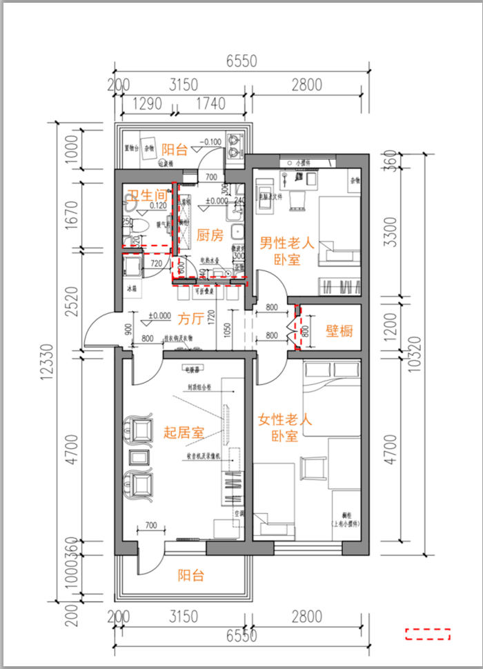
01-改造前平面布置 (带尺寸)
