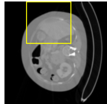
NMAR
