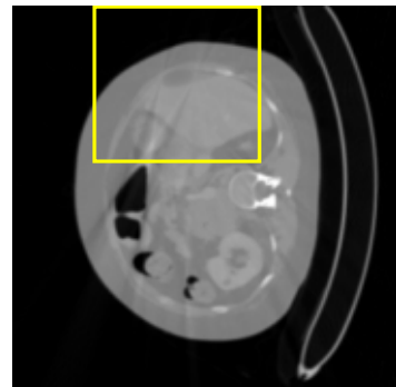
LI-MAR
