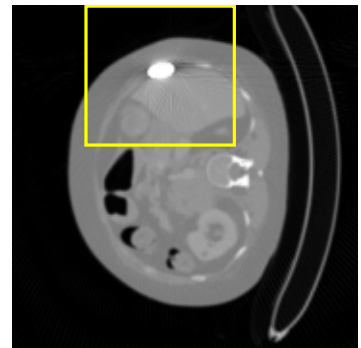
FBP
