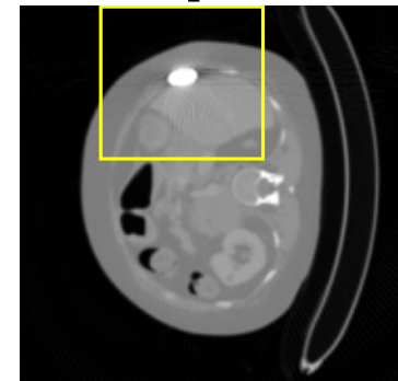
Input
