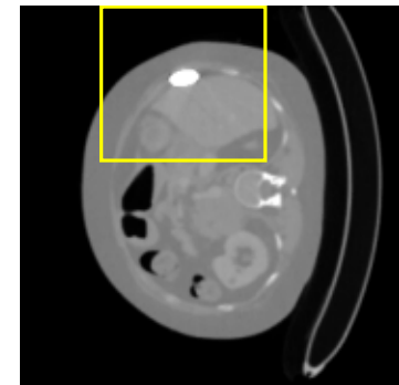
Ours
