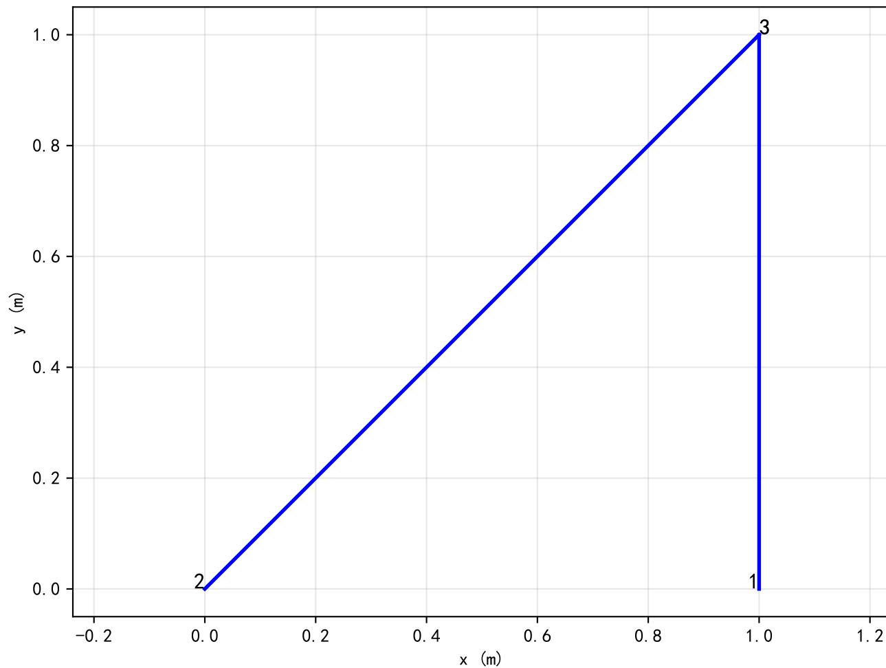
二维两杆桁架结构
