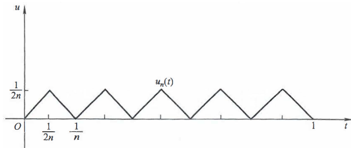
图 2.4: 锯齿形极小化序列 u_n
