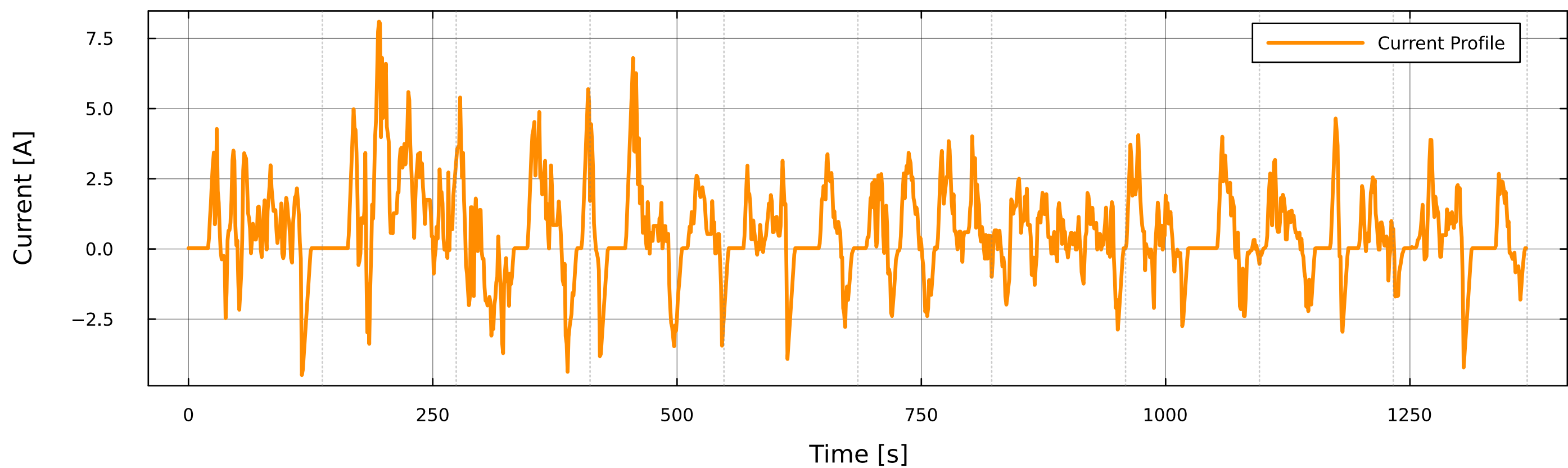
UDDS Current Profile
