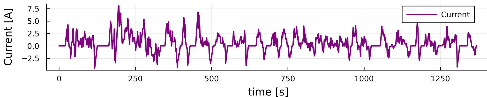
UDDS Current Profile
