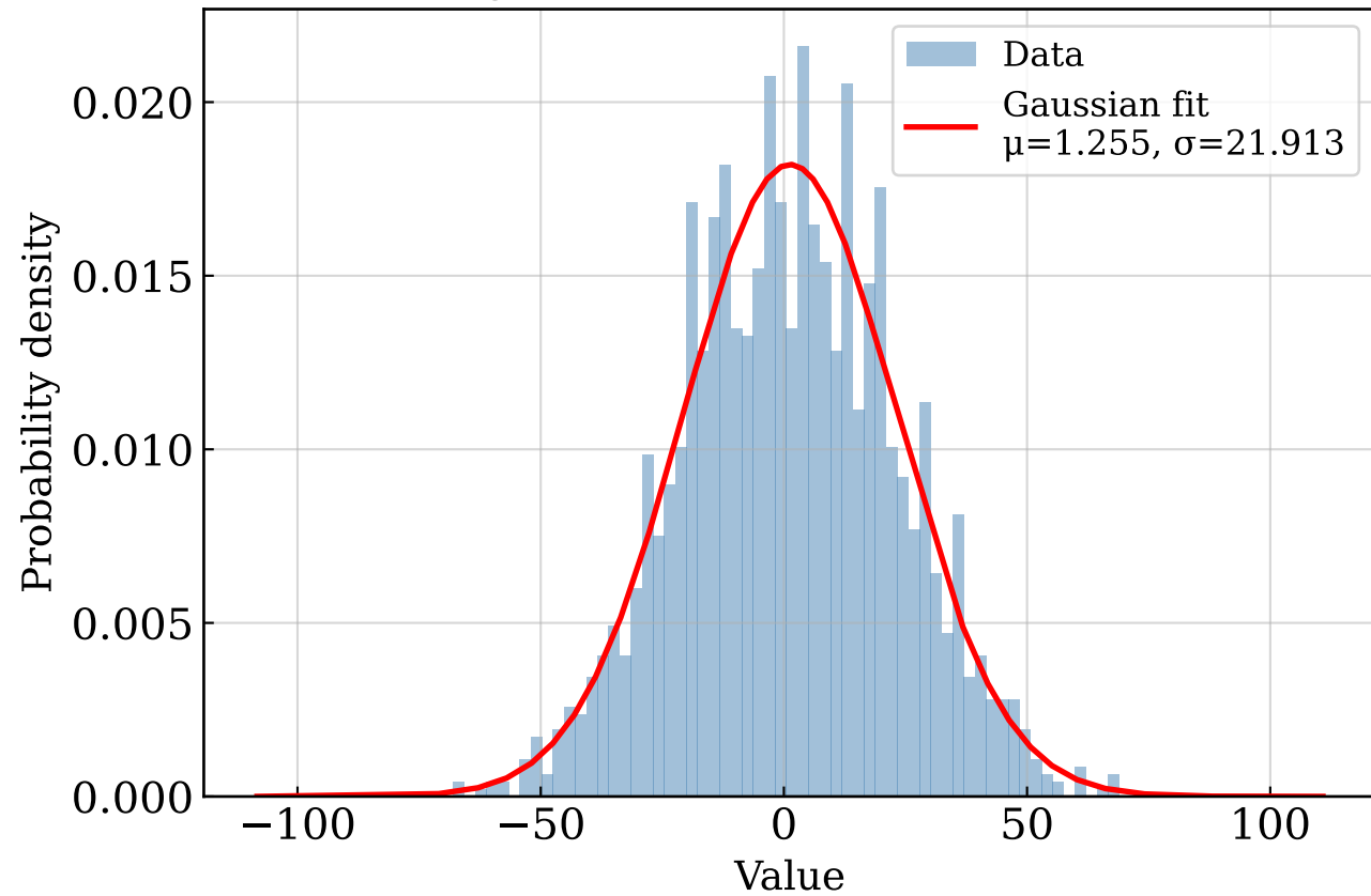
Histogram vs Gaussian (kurtosis=-0.1978)
