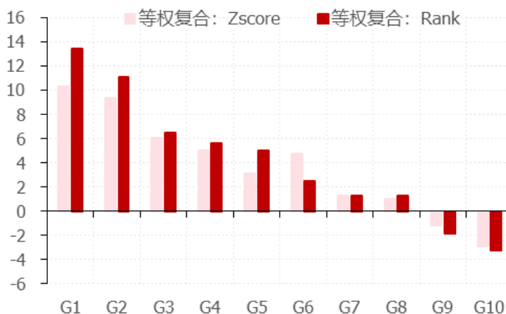
复合因子分组超额收益 (%)
