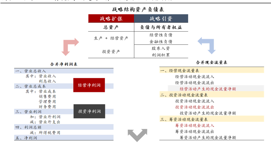
图表 1. 基于企业业务类型，构建更纯粹、不易操纵的财报指标
