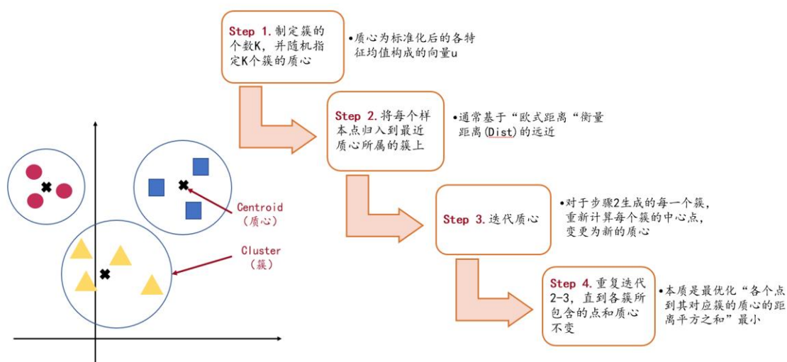
图表 8. K-Means 算法原理
