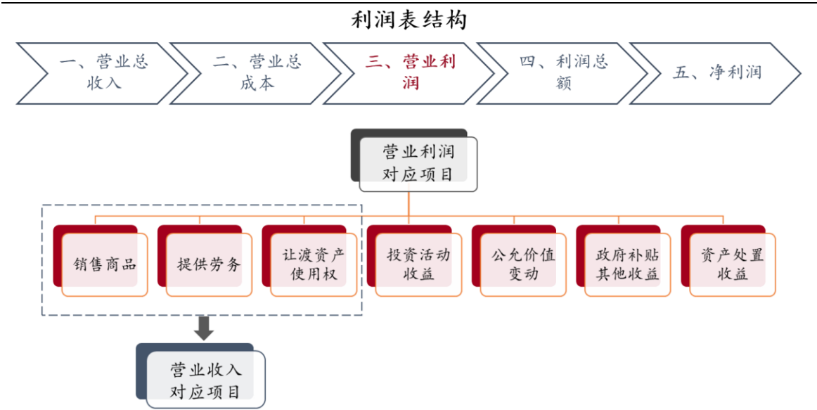
图表 2. 营业利润项目口径不够“纯粹”
