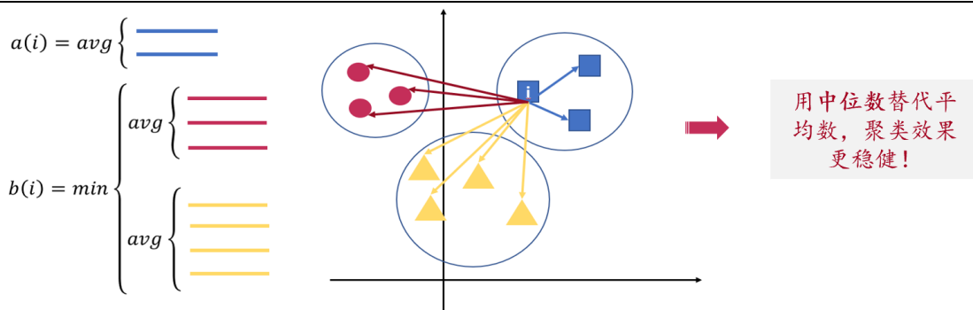
图表 10. 基于簇内中位数构建的轮廓系数，其聚类效果更为稳健
