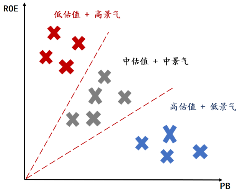
图表 6. 结合基本面与 A 股市场定价的因子中性化思想
