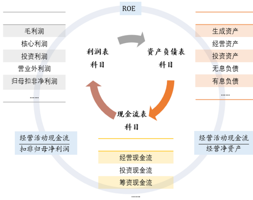
图表 4. 基于“跨报表验证”思路构建指标
