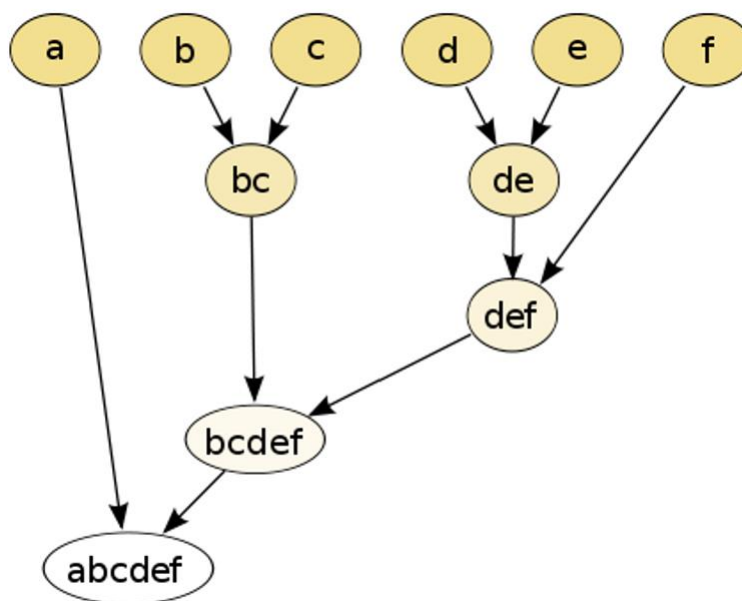
图表 9. “自下而上”的凝聚层次聚类方法
