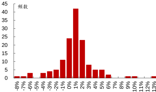
图表29: turn_6m 因子分层组合 1 相对沪深 300 月超额收益分布图
