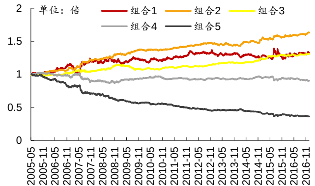
图表60: std_turn_1m 因子各层组合净值除以基准组合净值示意图
