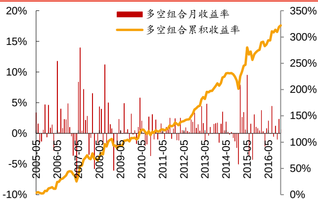
图表46: bias_turn_3m 因子多空组合月收益率及累积收益率
