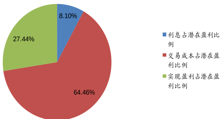
图 19: 实证结果之利润构成分析 (融资融券利息 5%, 交易成本双边 0.2%)
