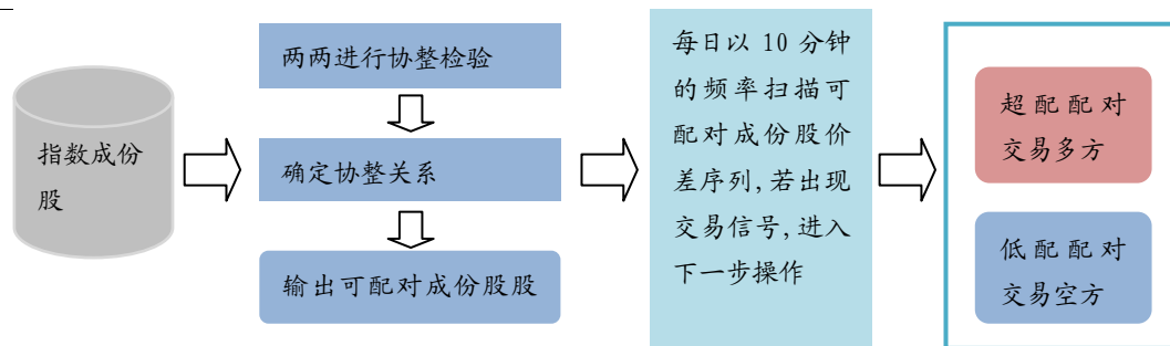
图 6：配对交易指数增强流程
