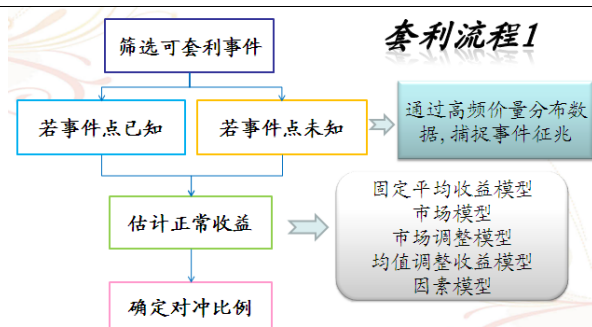
图 1：事件套利流程 1
