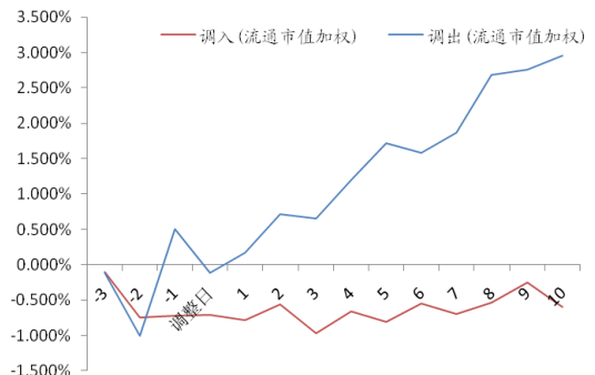
图 14: 调整日前后调入调出成份股票累积异常收益率变化
