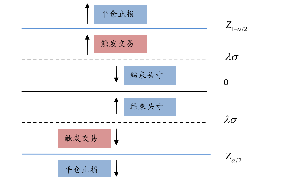
图 3：配对交易触发止损示意图
