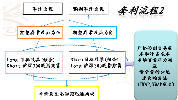
图 2：事件套利流程 2
