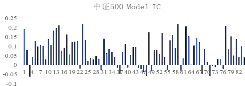
图：中证 500 Model IC 序列
