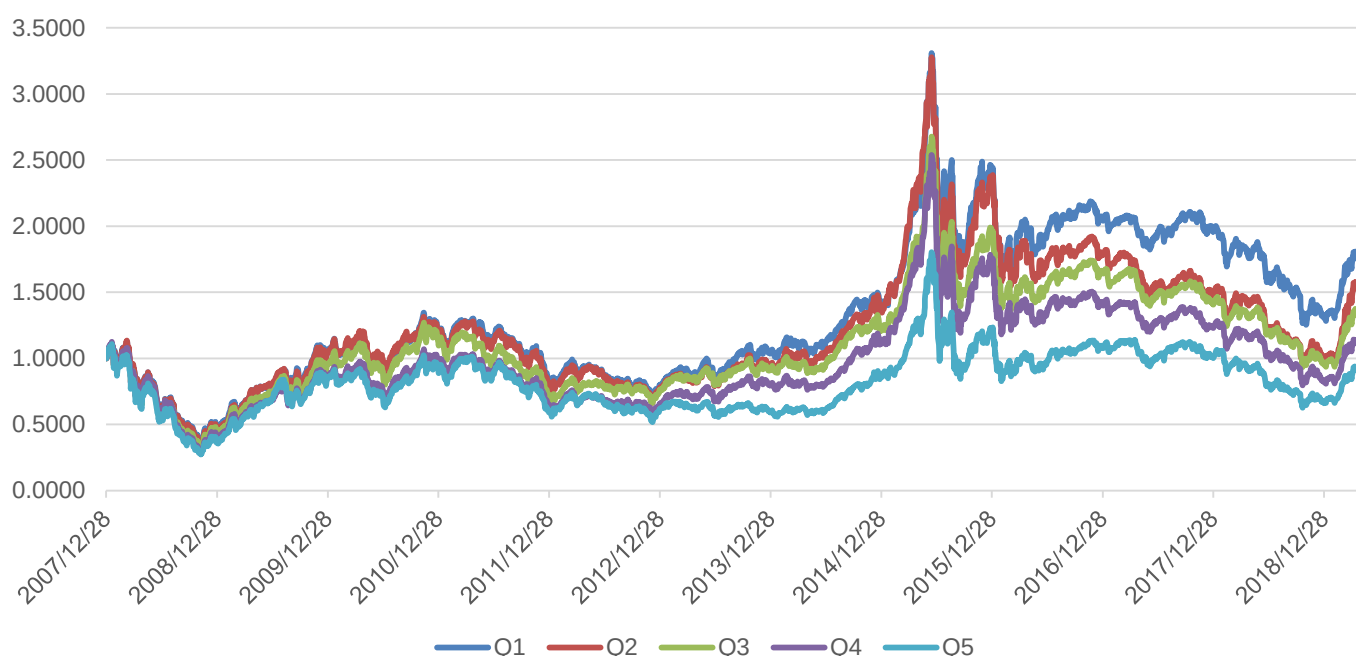
图19：中证500内情绪Beta因子5档回测（Q1低情绪Beta，Q5高情绪Beta）
