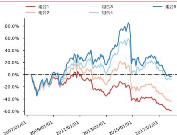
图 128 Tech_skew_1m 分层组合走势图（上证 50）
