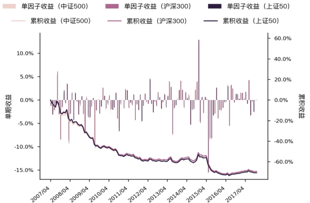
图 87 Tech_rsi_24d 单因子单期收益与累积收益图 (WLS)
