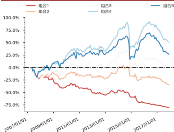
图 79 Tech_rsi_24d 分层组合走势图 (沪深 300)
