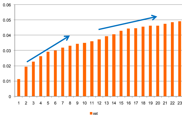
图 6 持有期平均收益率
