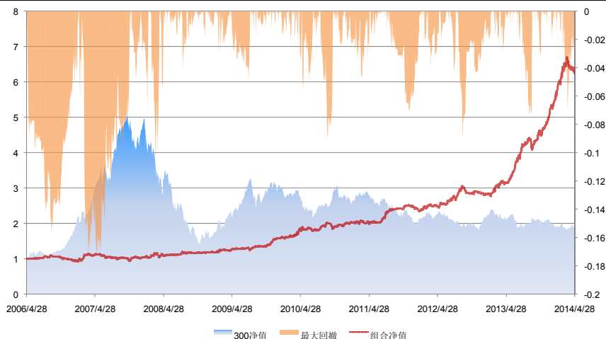
图 8 组合净值表现（2006-2014）
