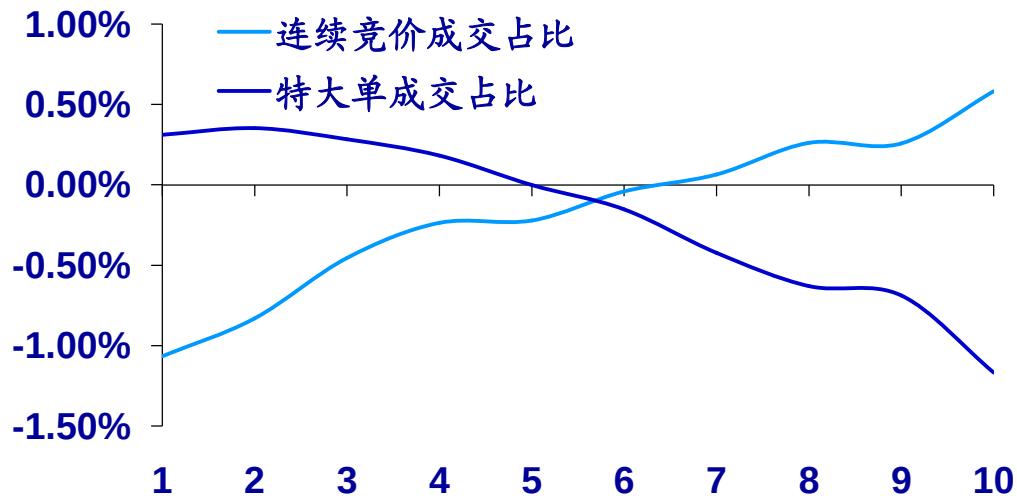
图：成交占比类因子回归残差选股的横截面效果
