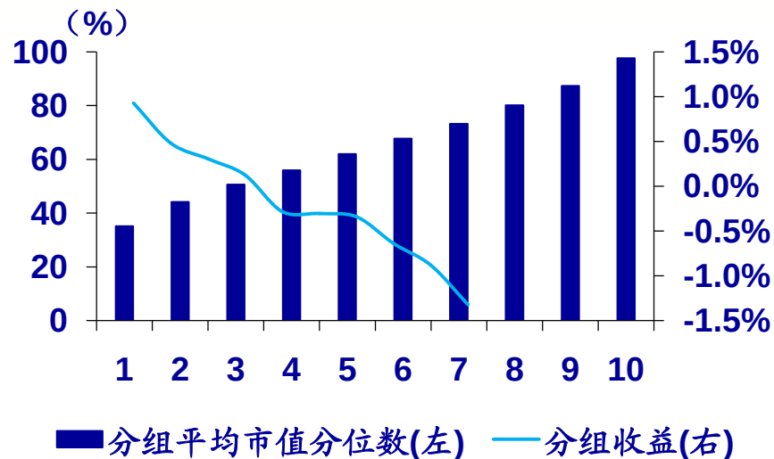
图：特大单成交占比因子的市值风格特征
