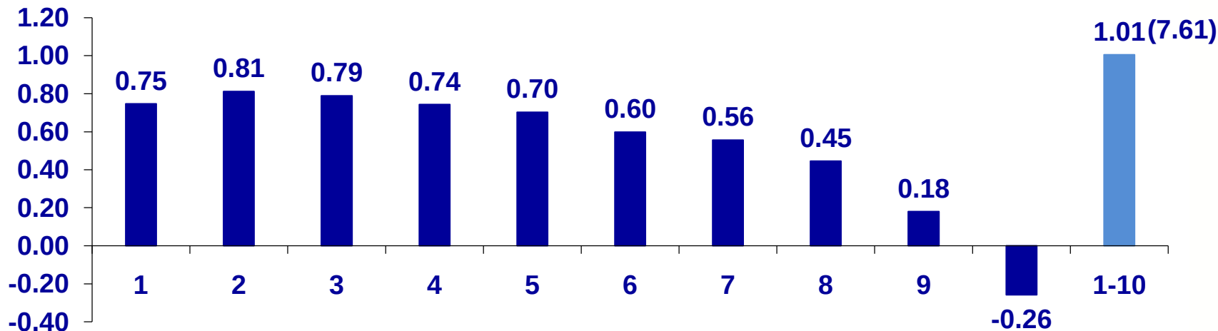
图：已实现偏度因子选股的横截面效果（%）
