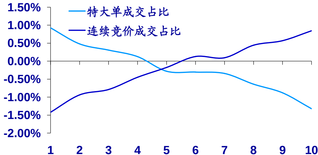
图：成交占比类因子选股的横截面效果
