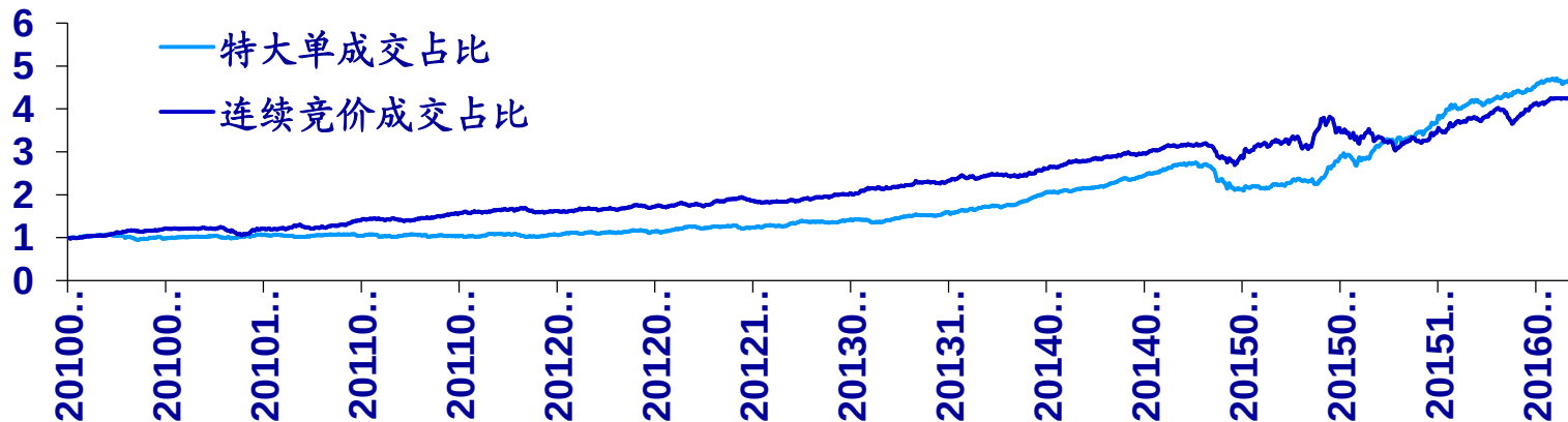
图：成交占比类因子选股的累计净值
