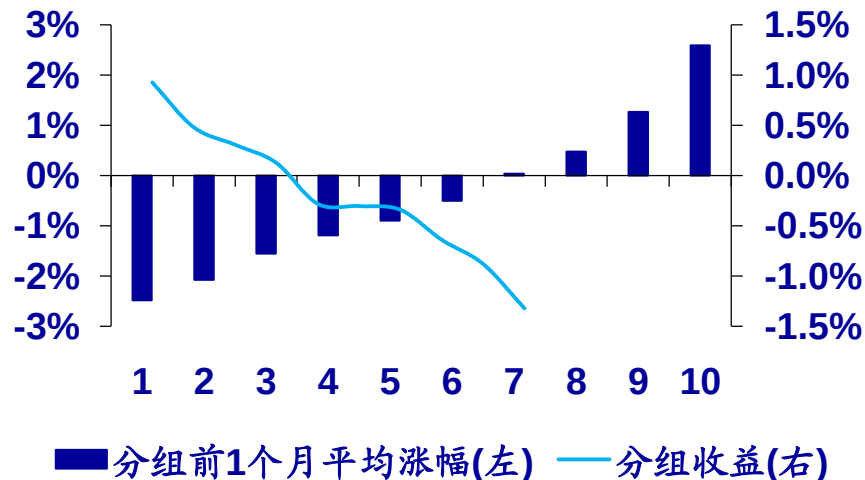
图：特大单成交占比因子的反转风格特征
