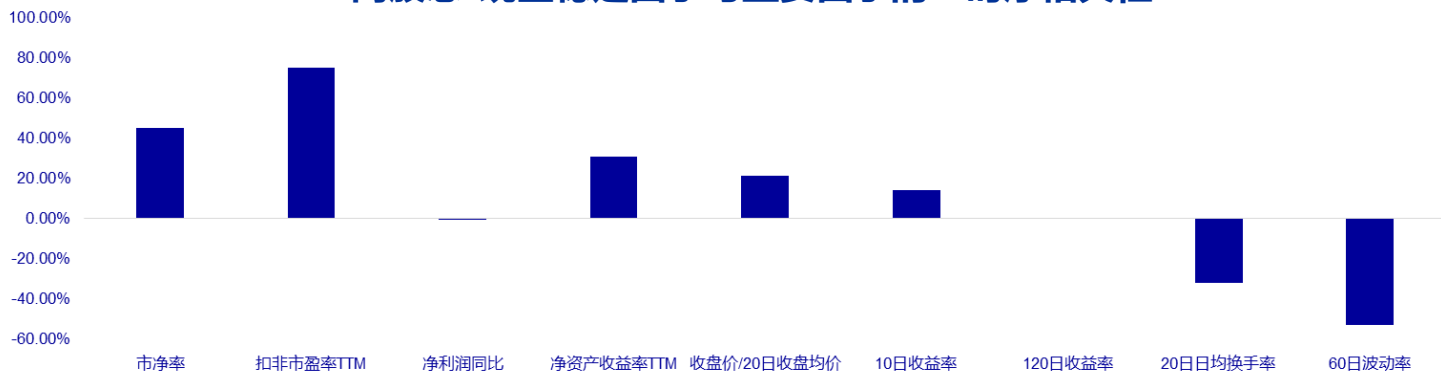
高股息-现金稳定因子与主要因子的IC时序相关性
