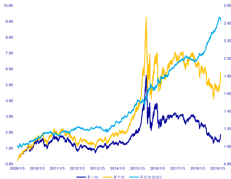
剔除相关性的高股息-现金稳定因子多空净值
