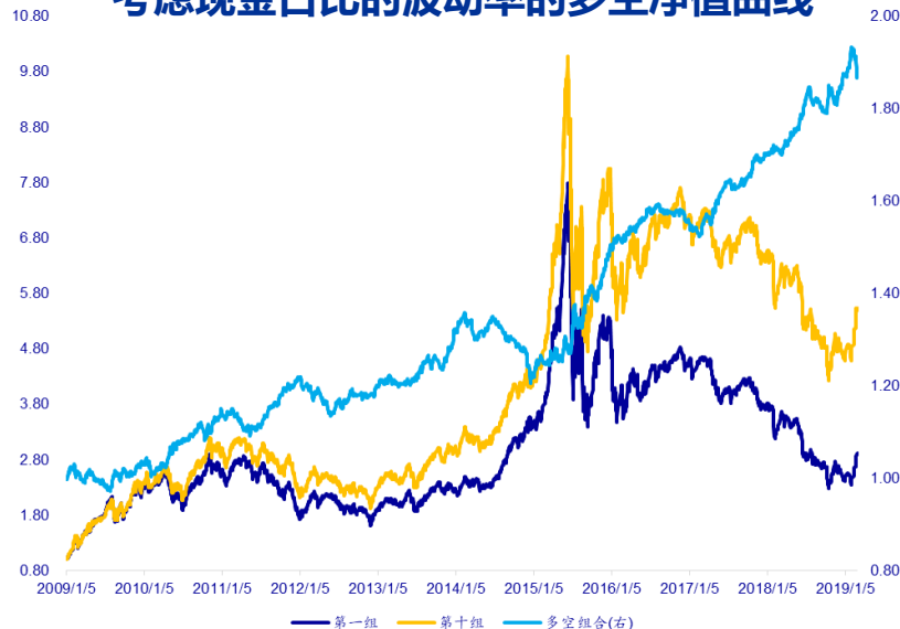
考虑现金占比的波动率的多空净值曲线
