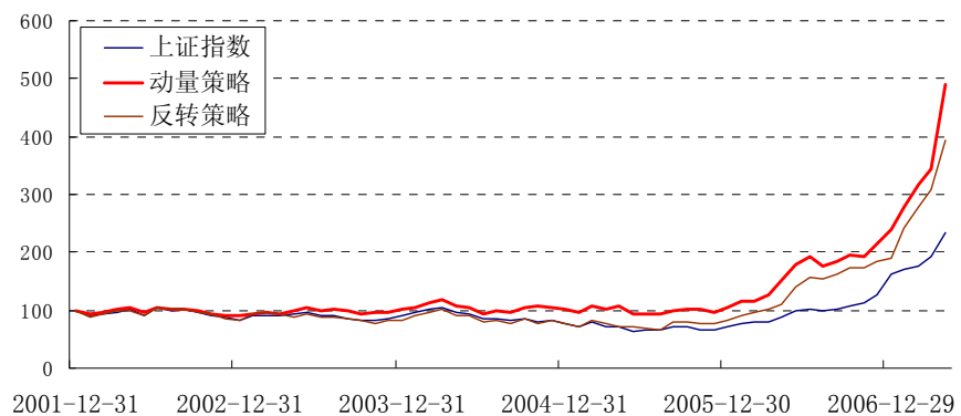
图 9、股票价格动量反转策略的模拟投资组合走势 2002.1-2007.4
