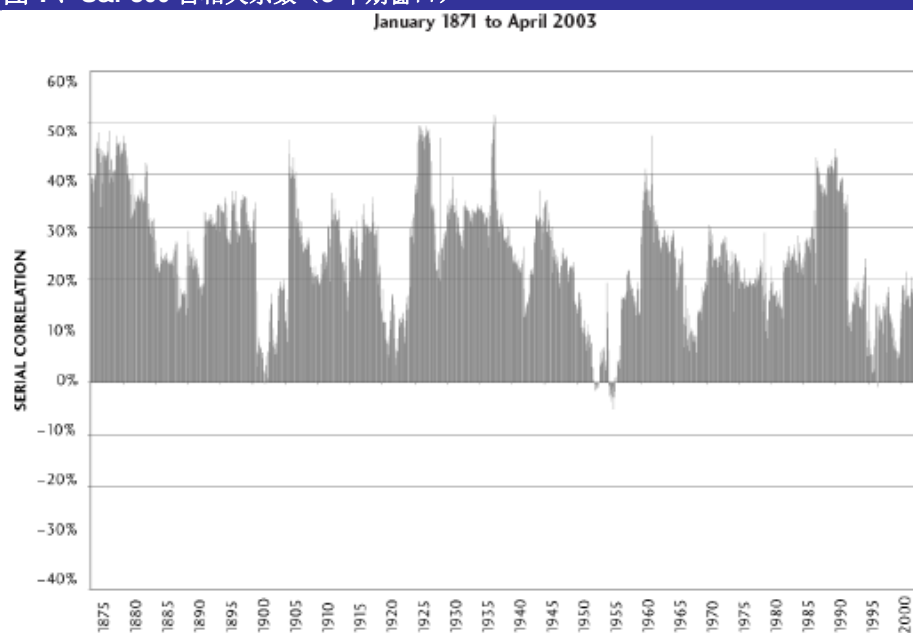
图 7、S&P500 自相关系数 (5 年期窗口)
