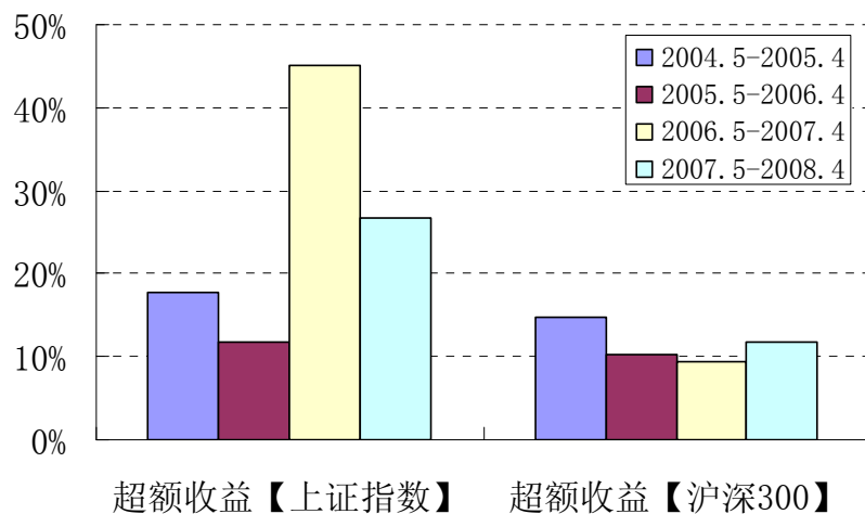
图 6、G50 投资组合的超额收益水平（2004.5.10-2008.4.30）
