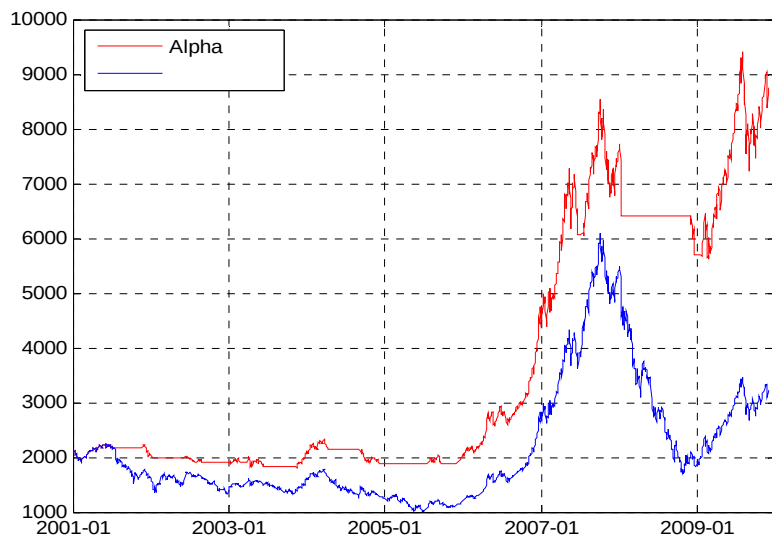
图 12 应用于上证综指的策略业绩表现 11
