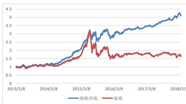
图 16：策略净值
