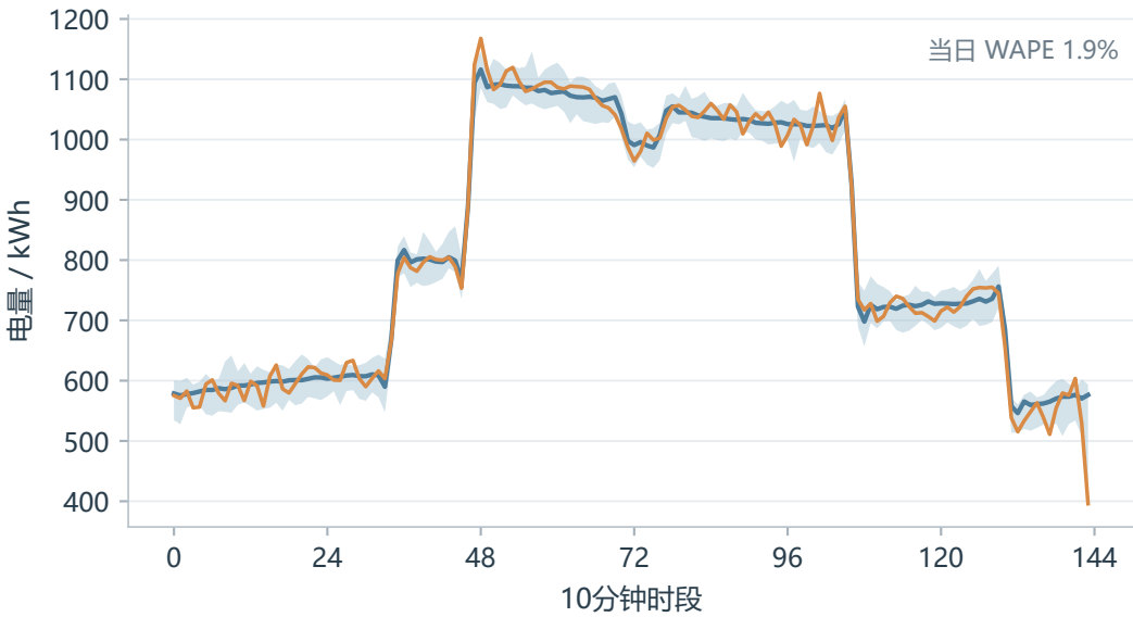
2025-11-20 负荷
