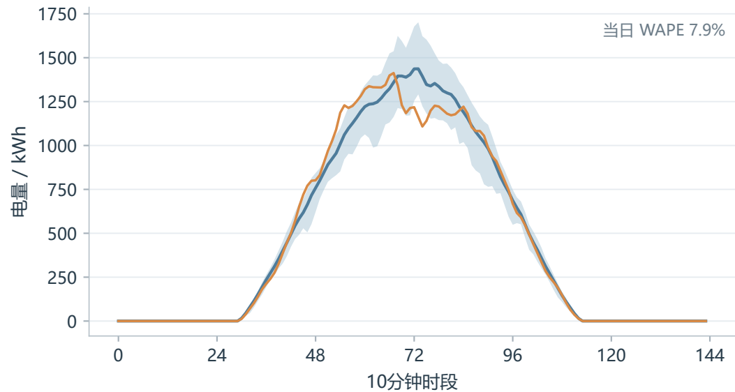
2025-11-20 光伏
