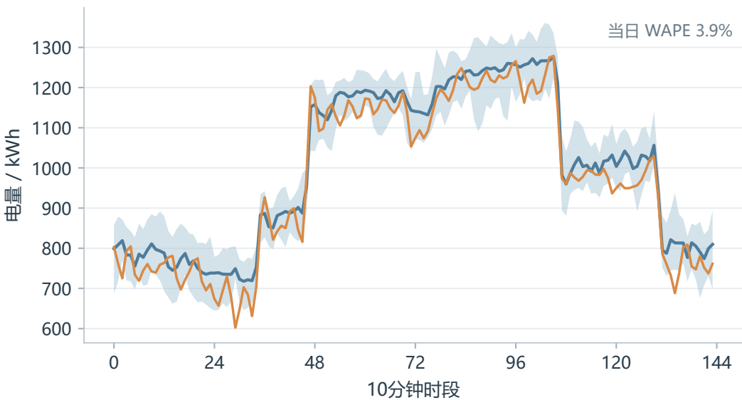
2025-11-20 负荷
