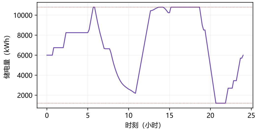
储能 SOC 轨迹 (虚线为上下限)
