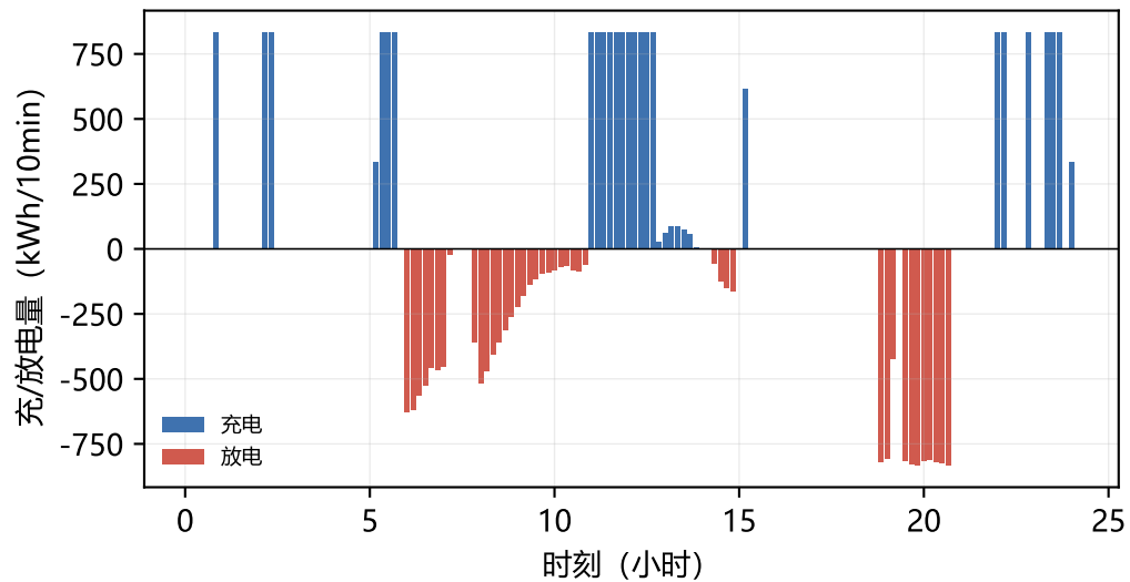
储能充放电 (负值为放电)
