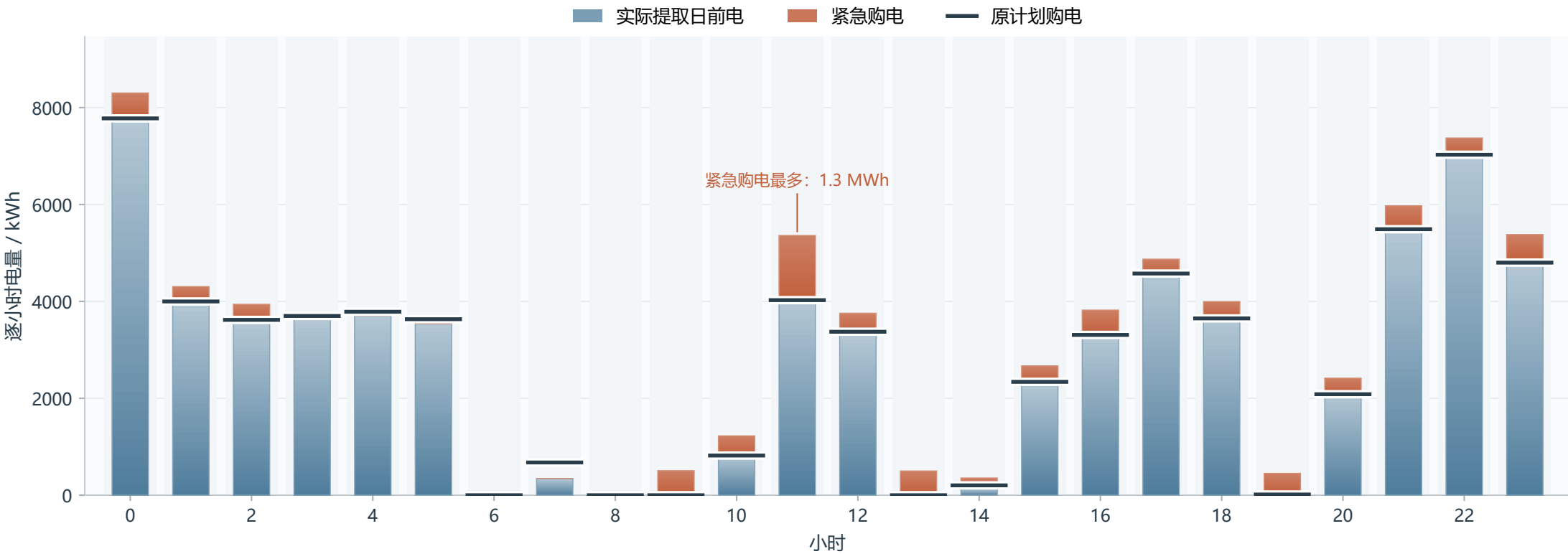
2025-06-01 逐小时购电结构：计划 68.9 MWh，另需紧急购电 8.4 MWh (+12%)
