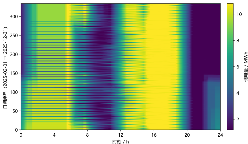
图 13 全年储电量分布（日期 × 时刻）
