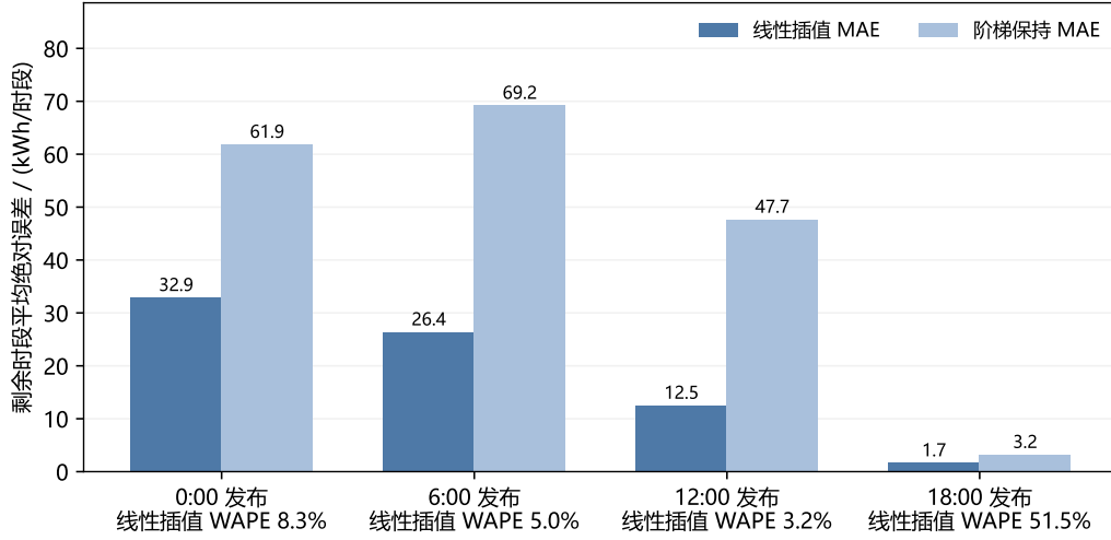
图 8 四个发布时刻的预报转换误差（线性插值 vs 阶梯保持）
