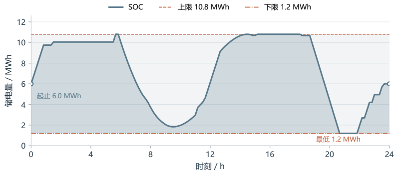
图 6 全天储电量变化及运行边界
