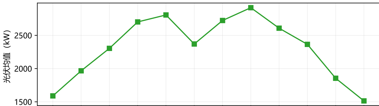
(b) 光伏功率月均值
