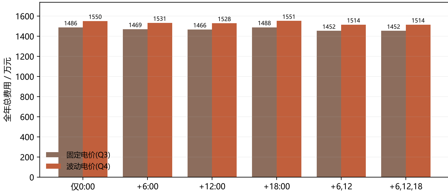
波动电价 vs 固定电价：六种更新策略全年费用
