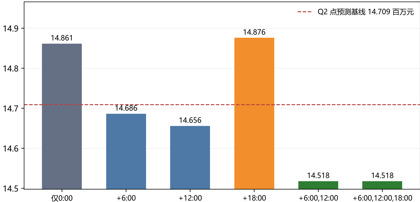
全年实际购电费用 / 百万元
