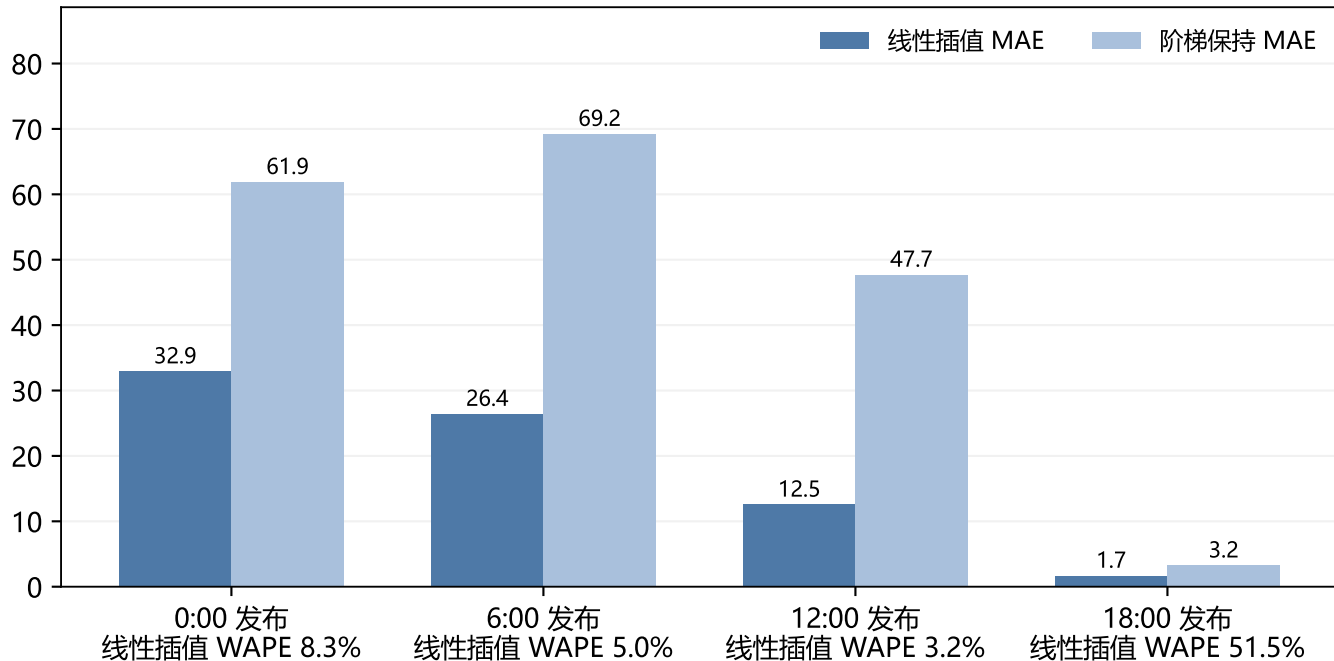
剩余时段平均绝对误差 / (kWh/时段)
