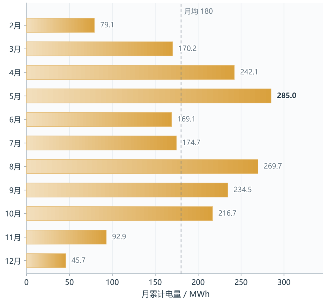
弃光：光伏出力无法消纳
