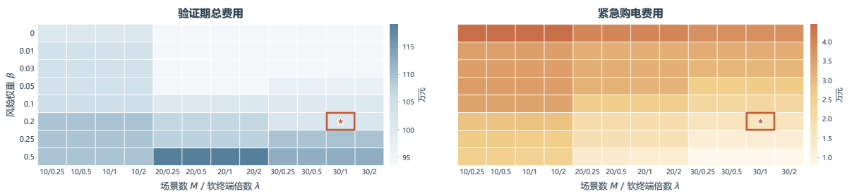
图 9 验证期候选参数的费用与风险分布
