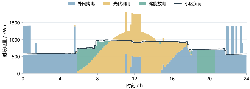
图 5 全天购电与储能充放电调度
