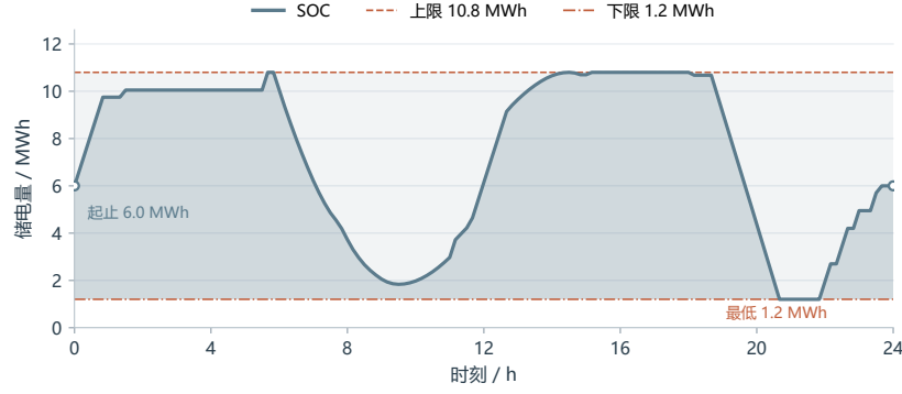
图 6 全天储电量变化及运行边界
