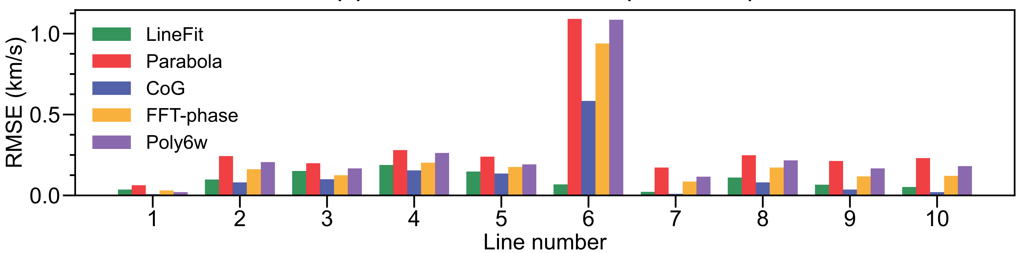
(d) Per-line RMSE vs truth (all 10 lines)
