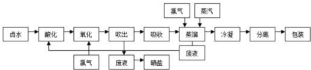
海化股份溴产品生产工艺流程图
