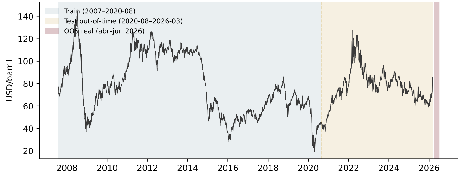
Brent (FRED DCOILBRENTU) y particiones temporales de la evaluación
