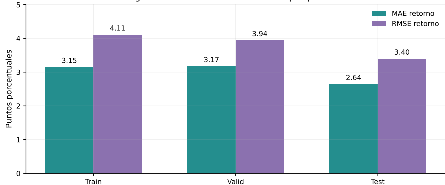
Regresión del retorno a 1 día: error por partición
