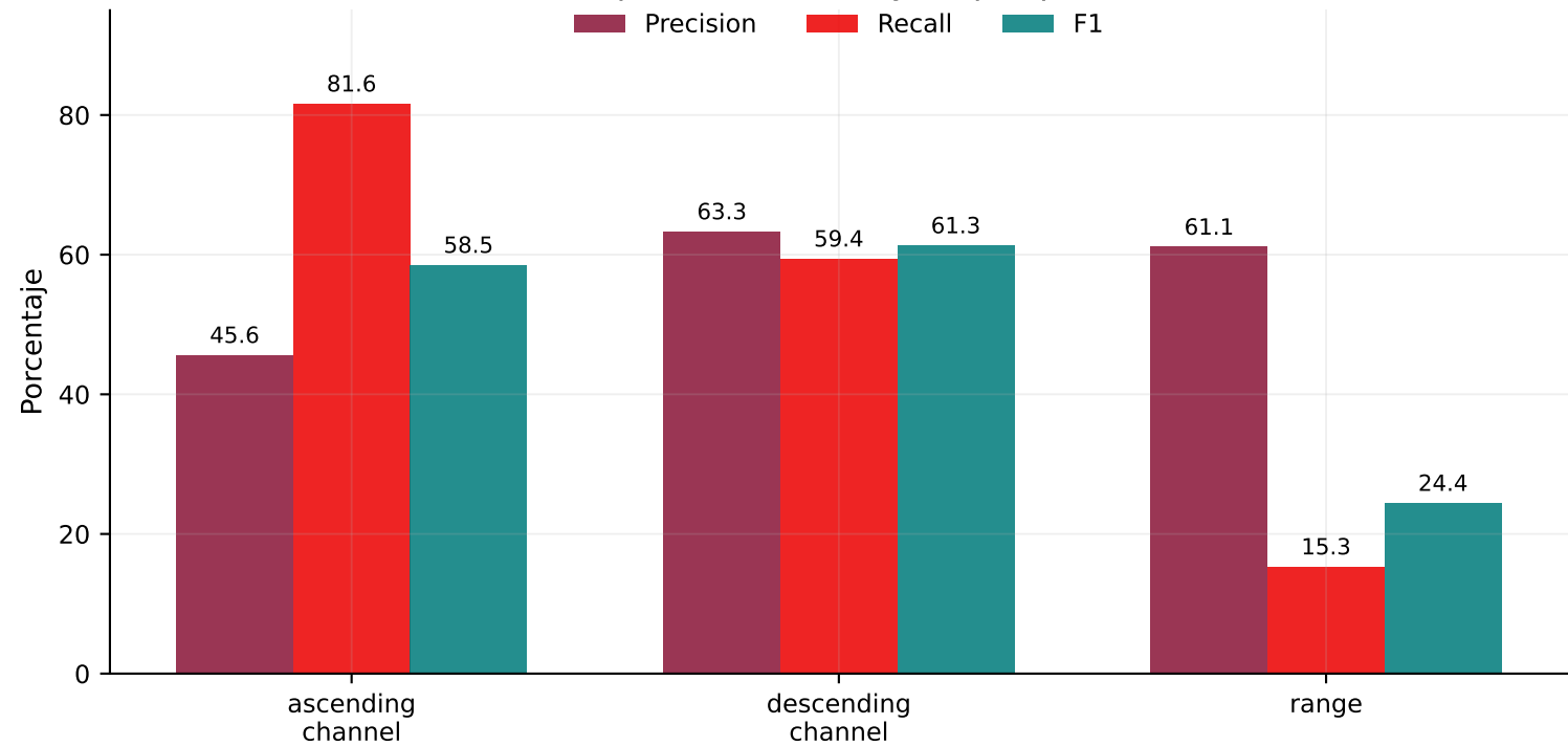
Test: precision, recall y F1 por patrón
