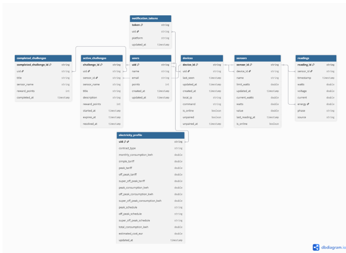
Figura 11- Diagrama ER
