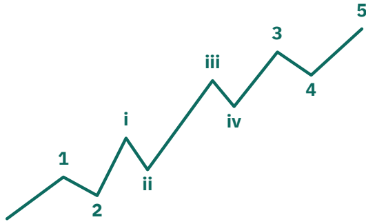
الموجة 3 ممتدة
