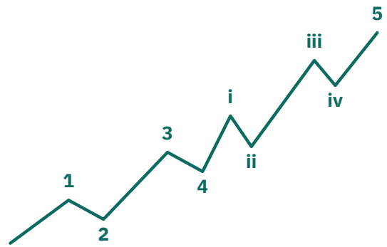
الموجة 5 ممتدة
