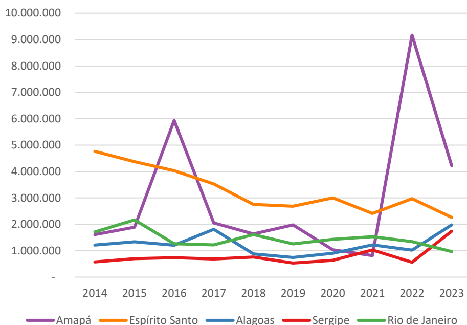
Gráfico 4. Emissões de CO 2 e (t) GWP-AR5 em mudança de uso da terra e floresta dos 5 estados que tiveram a menor emissão em 2023
