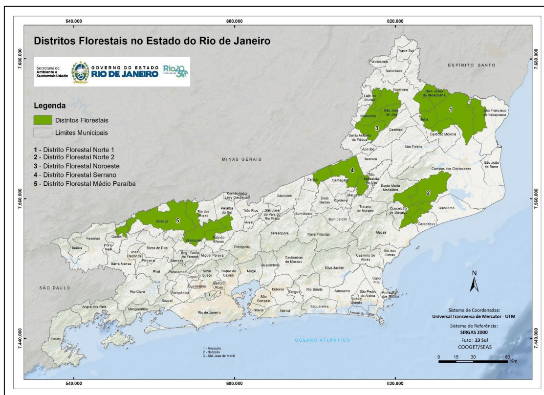
Figura 3 – Distritos Florestais do estado do Rio de Janeiro
