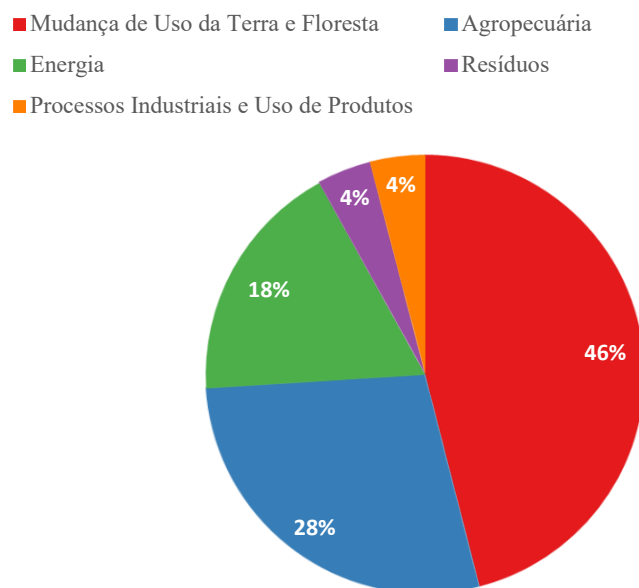
Gráfico 1. Participação (%) dos setores no perfil das emissões brasileiras de gases de efeito estufa em 2023
