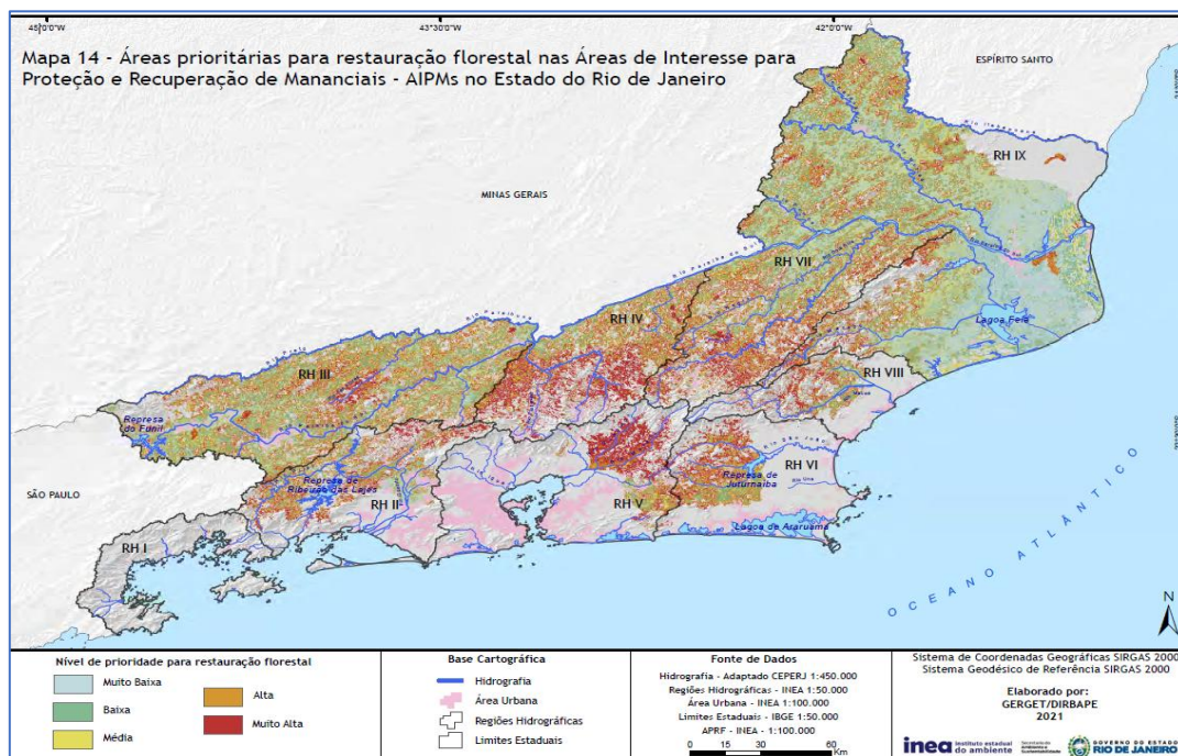
Figura 2 – Áreas prioritárias para restauração florestal nas Áreas de Interesse para Proteção e Recuperação de mananciais no ERJ
