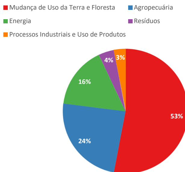
Gráfico 2. Participação (%) dos setores no perfil das emissões brasileiras de gases de efeito estufa em 2022
