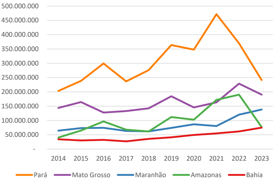
Gráfico 3. Emissões de CO 2 e (t) GWP-AR5 em mudança de uso da terra e floresta dos 5 estados que tiveram a maior emissão em 2023
