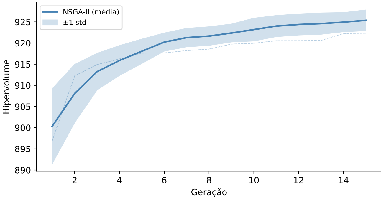
Convergência do Hipervolume — NSGA-II (10 sementes)
