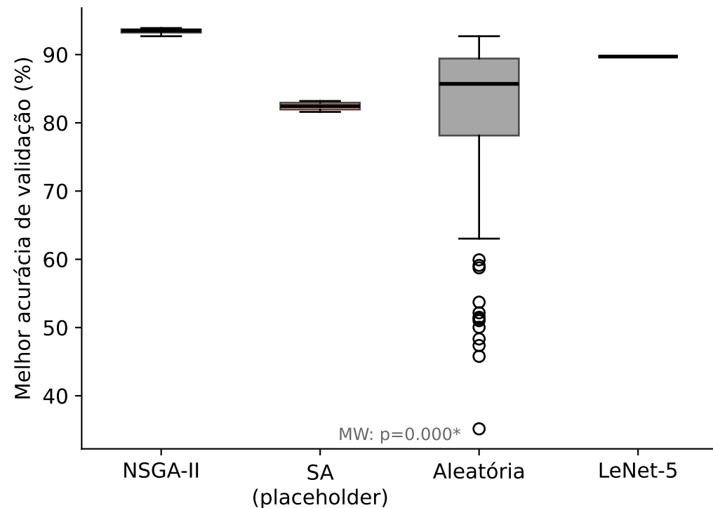
Distribuição da melhor acurácia (10 sementes)
